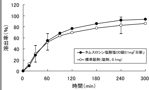
pH7.5 100回転
