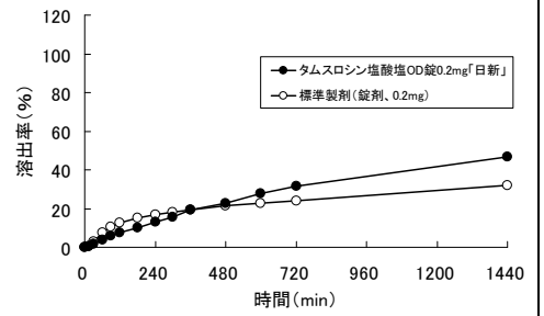
水 50回転
